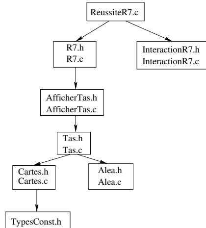
FIGURE 1 – Dépendances entre les fichiers C fournis
