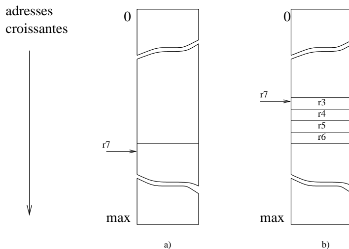
FIGURE 2.9 – Transfert multiples mémoire/registres : STMFd r7!, {r4,r5,r6} ou ( STMDB ... ) permet de passer de l'état a) de la mémoire à l'état b). LDMFD r7!, {r4,r5,r6} (ou LDMIA ... ) réalise l'inverse.
