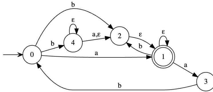
FIGURE 4 – Un ε-AEFND que l'on veut déterminer.
