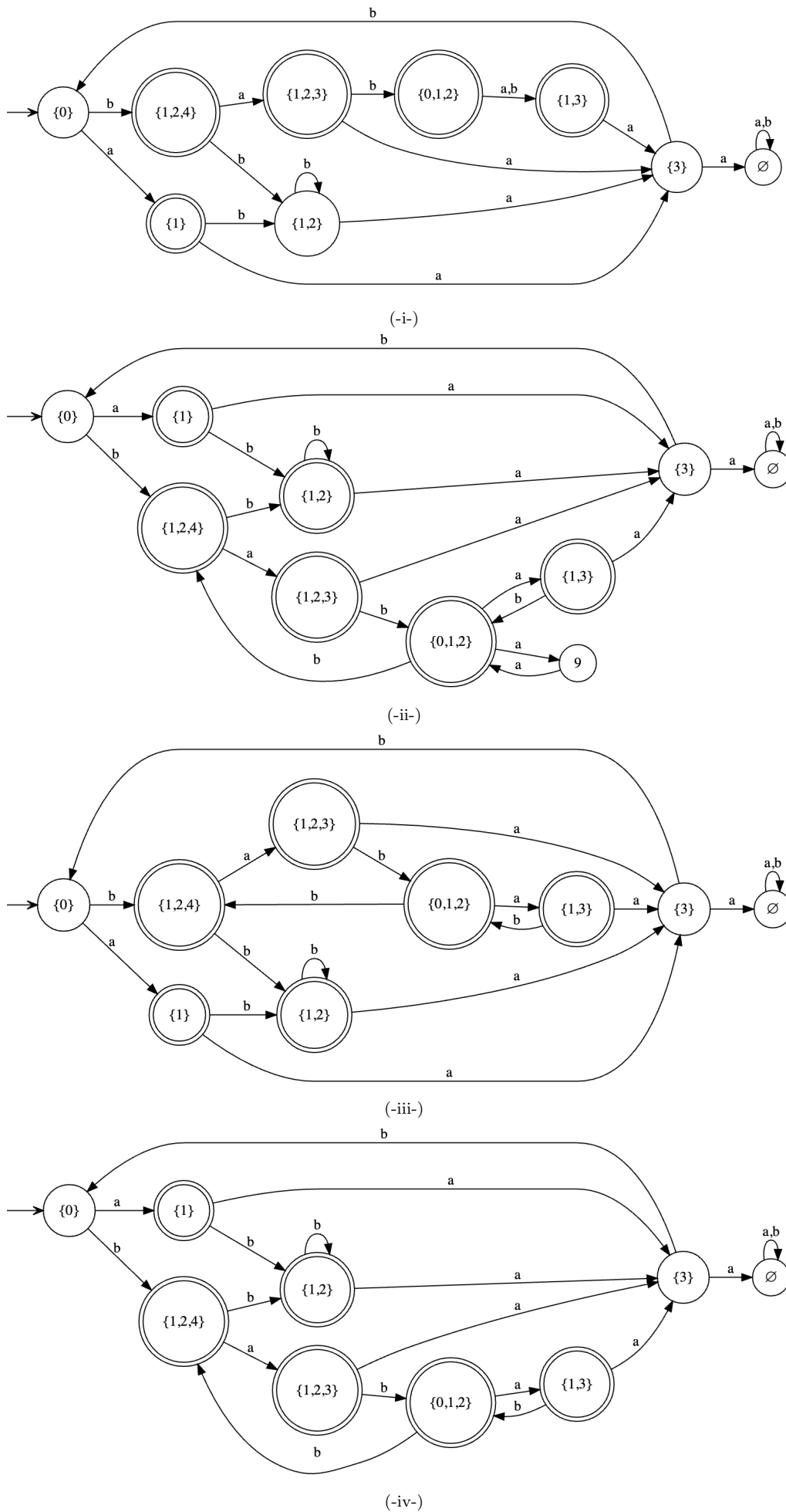
FIGURE 5 – Des automates résultant possiblement de l'algorithme de détermination.
