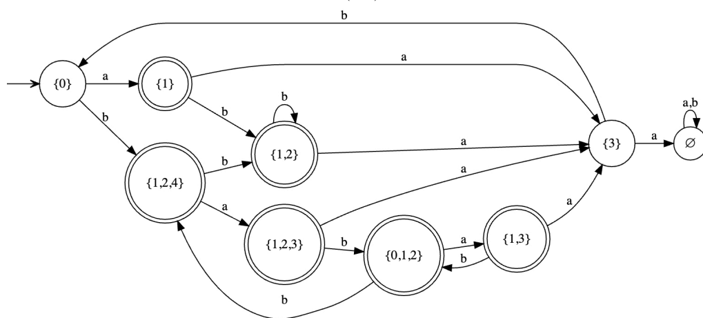
(IV) FIGURE 5 – Des automates résultant possiblement de l’algorithme de déterminisation.
