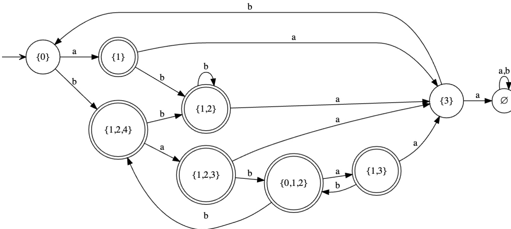
FIGURE 5 – Des automates résultant possiblement de l'algorithme de déterminisation.
