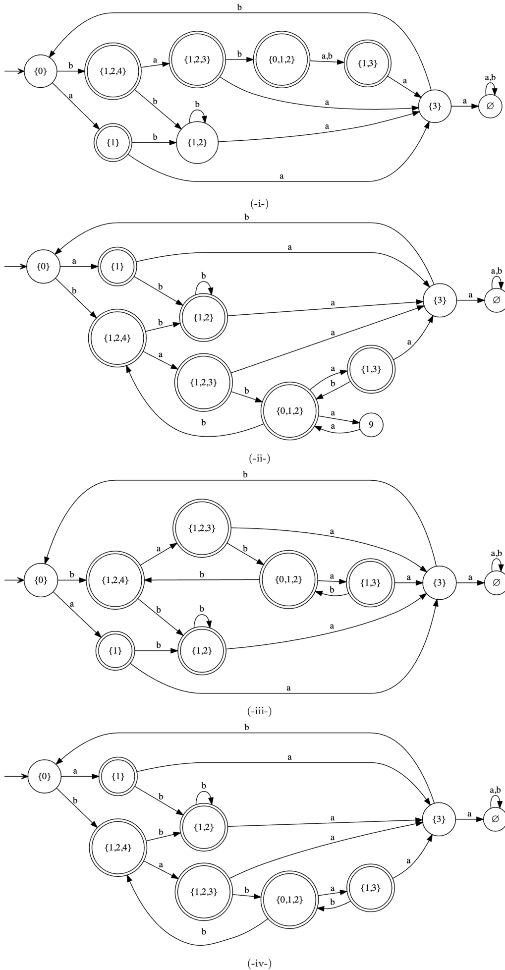
FIGURE 5 – Des automates résultant possiblement de l'algorithme de déterminisation.
