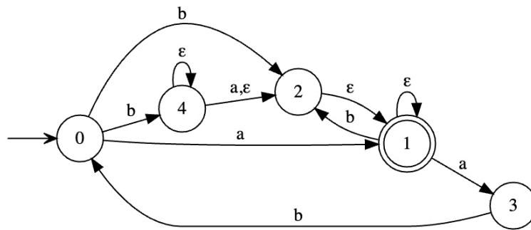
FIGURE 4 – Un ε-AEFD que l'on veut déterminer.
