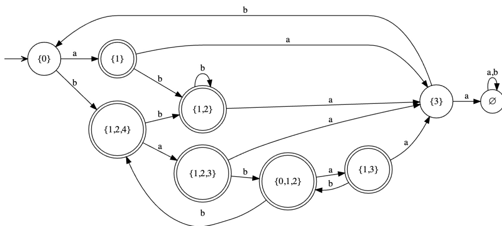
FIGURE 5 – Des automates résultant possiblement de l'algorithme de détermination.
