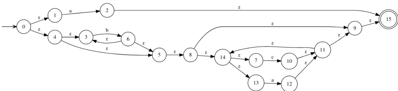
FIGURE 5 – Des automates résultant possiblement de la traduction compositionnelle d'expressions régulières vers \epsilon -AEFND, pour l'expression (a + b^* \cdot (c + a)^*) .
